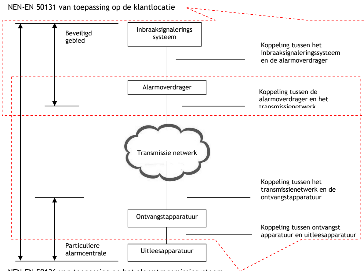
Figuur 1 schematische weergave relatie tussen de NEN-EN 50131 en NEN-EN 50136
